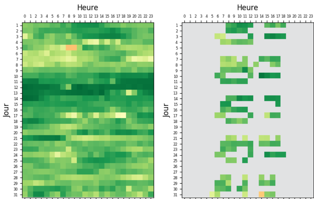
Fig 4 - PM10 en concentration horaire en \mu\text{g}/\text{m}^3 sur le mois de Mars pour les capteurs fixes (à gauche) et les capteurs mobiles (à droite)
