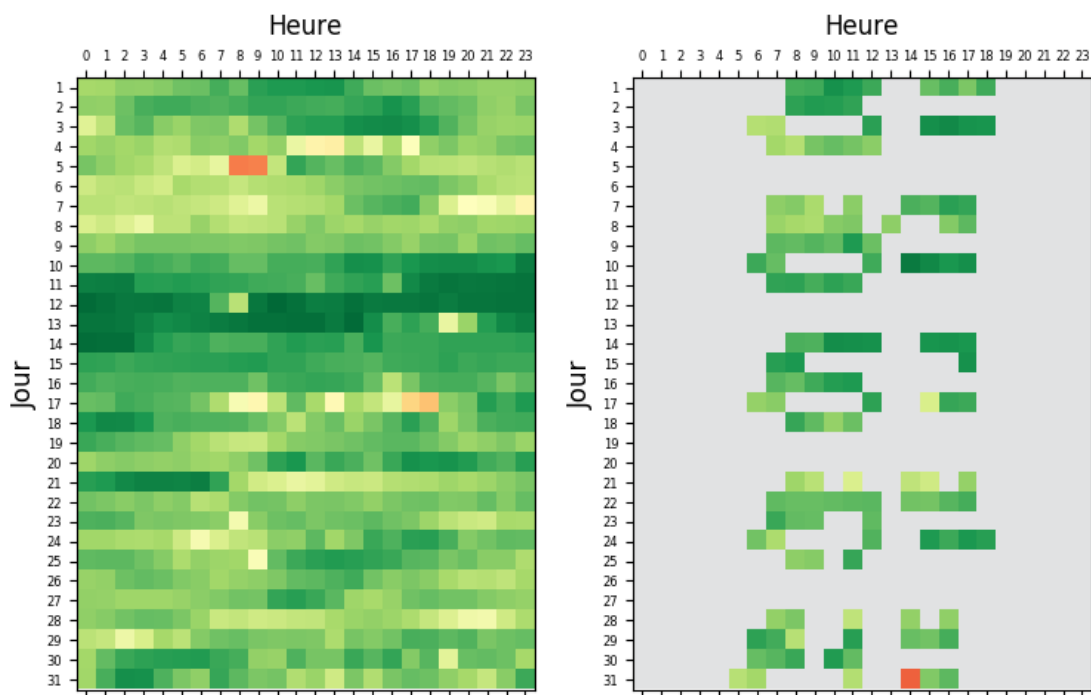
Fig 2 - PM2.5 en concentration horaire en µg/m 3 sur le mois de Mars pour les capteurs fixes (à gauche) et les capteurs mobiles (à droite)
